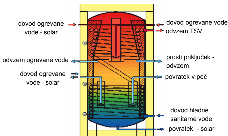
shema priključkov zalogovnika Quadro DU
