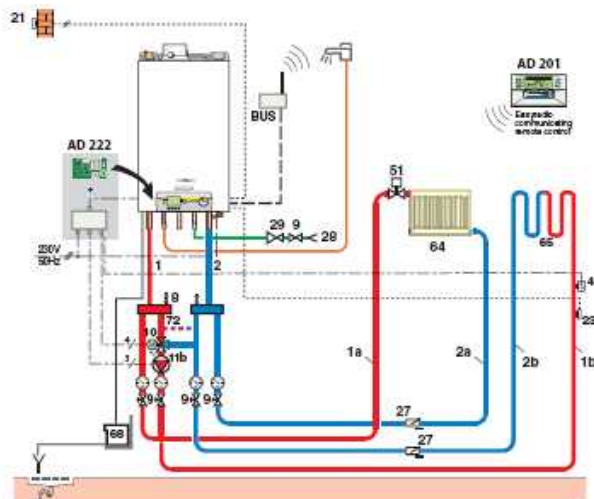
Primer hidravlične povezave kondenzacijskega kotla MCR MI s pretočnim ogrevanjem sanitarne vode z enim direktnim in enim mešalnim ogrevalnim krogom ter vremensko vodeno regulacijo
