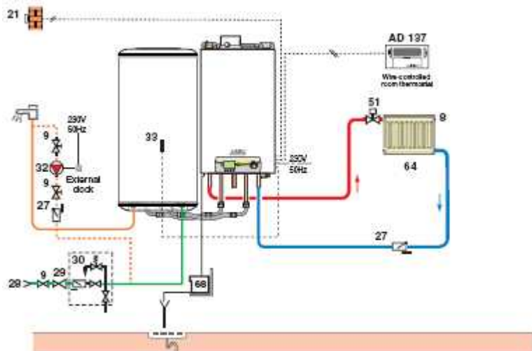
Primer hidravlične povezave kondenzacijskega kotla MCR24 z BMR80 grelnikom sanitarne vode, enim direktnim ogrevalnim krogom, zunanjim tipalom ter sobnim termostatom
