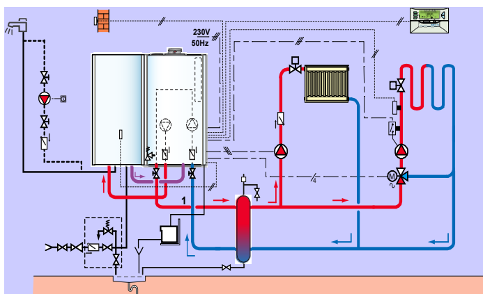
Primer hidravlične povezave kondenzacijskega kotla DPSM3 LP z grelnikom sanitarne vode z enim direktnim oziroma enim direktnim ter enim mešalnim sklopom preko hidravlične kretnice
