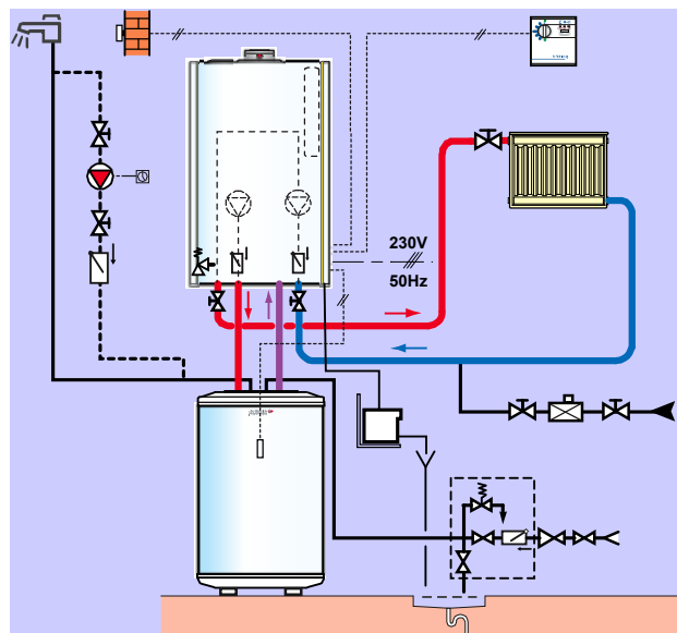
Vgradni mešalni sklop za DTG1300 - ELIDENS
